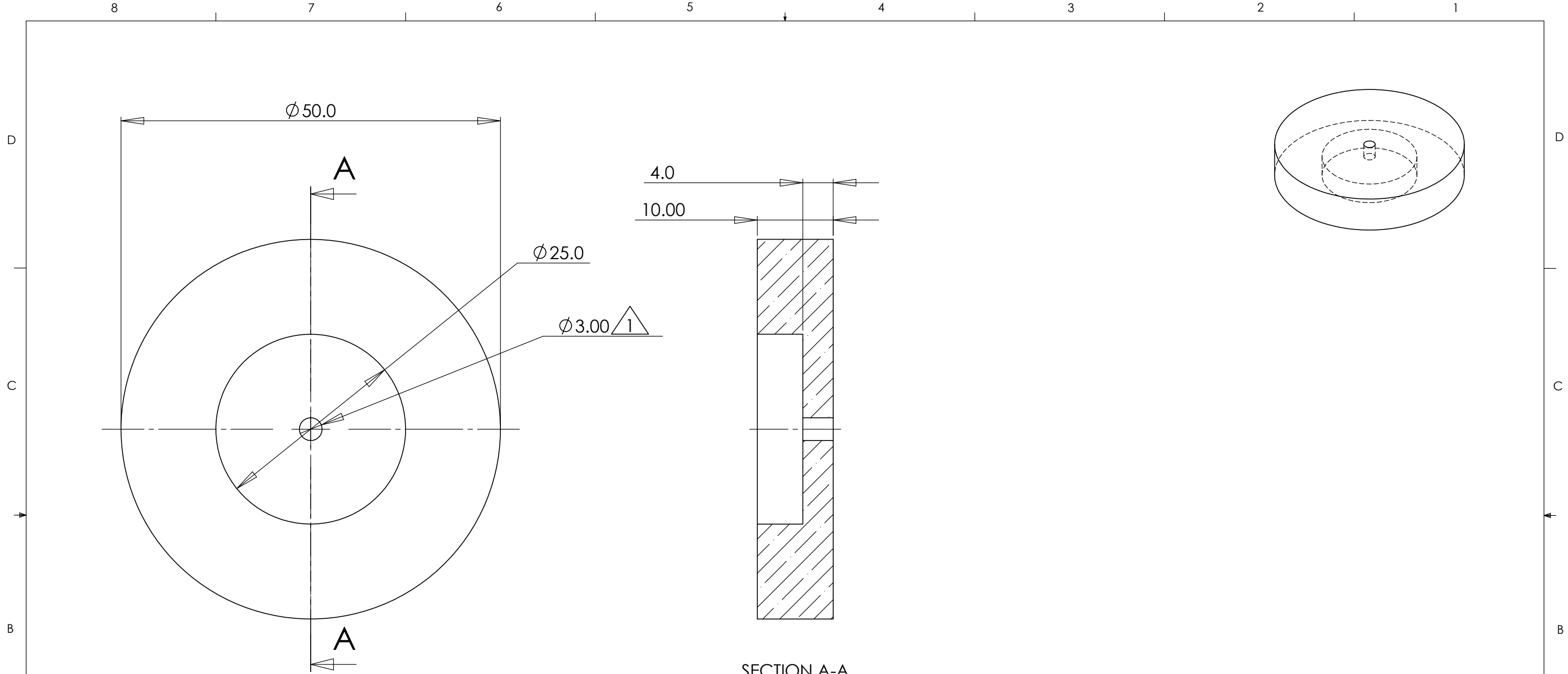
SECTION A-A
